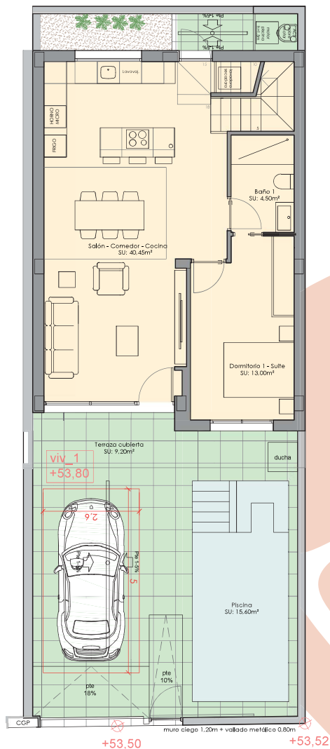
PLANTA BAJA
