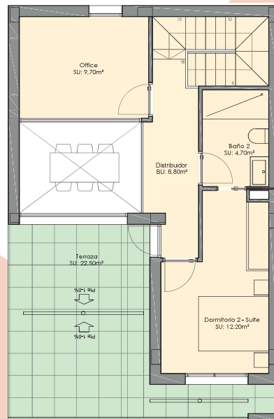
PLANTA PRIMERA
