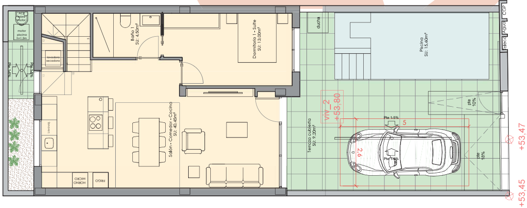
PLANTA BAJA
