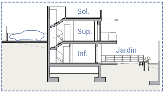
Sección / Section
