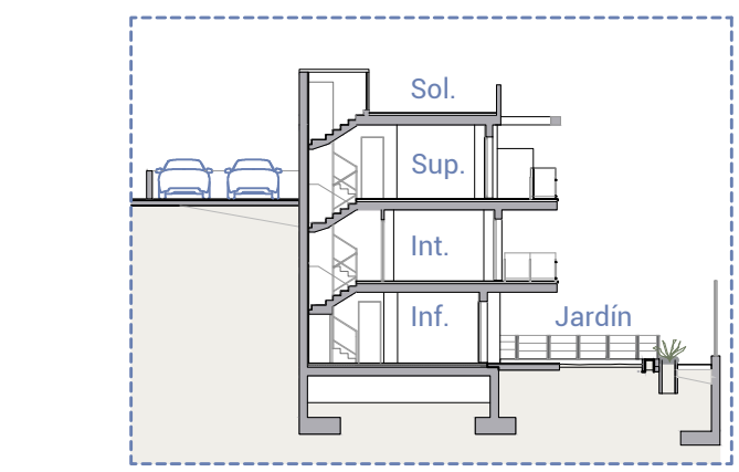
Sección / Section
