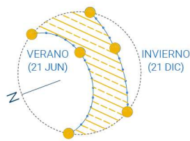
Soleamiento/Sunlight study
